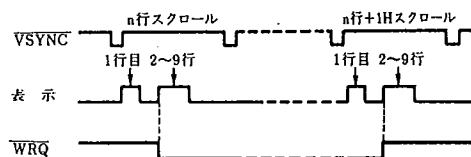
図 14 WRQ出力タイミング
