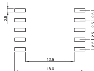
LAND PATTERNS(mm) 推奨ランド寸法
