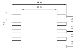
LAND PATTERNS(mm) 推奨ランド寸法
