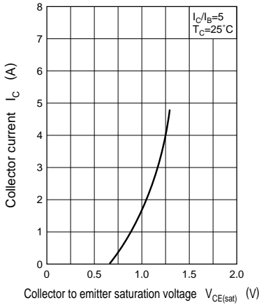
I_C - V_{CE(sat)}
