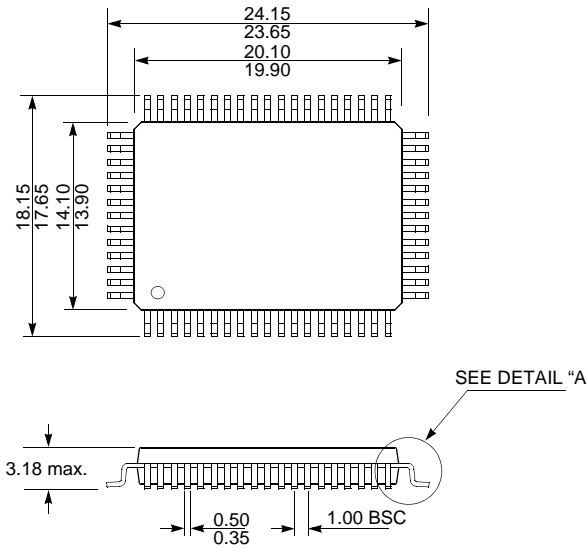
64MQFP
