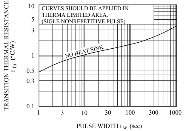
r_{th} - t_w
