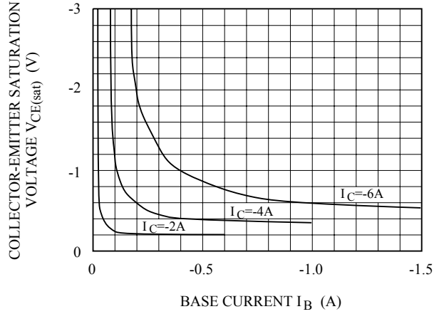
V_{CE(sat)} - I_B
