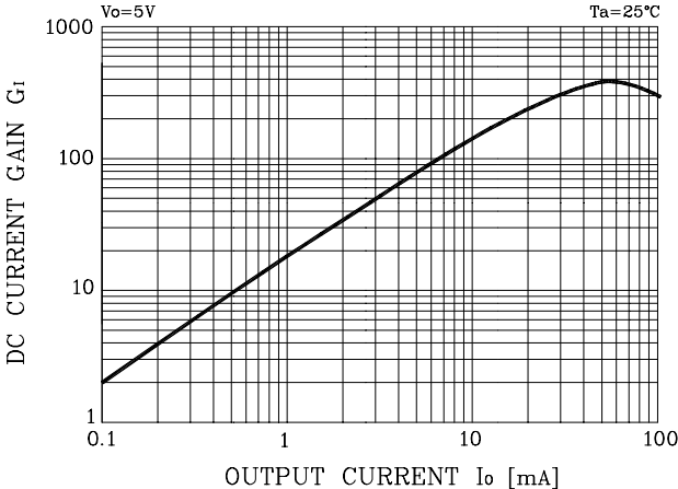
Fig. 3 G_I - I_o
