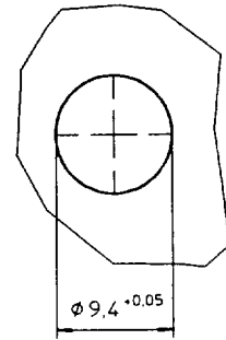
Einbauöffnung ohne O-Ring
