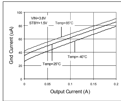
Fig. 187. IOUT - IIGND
