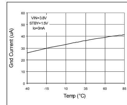
Fig. 193. IIGND - Temp
