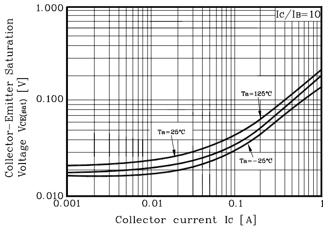
Fig. 3 V_{CE(sat)} - I_C
