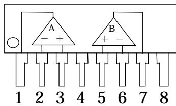
NJM14558L
