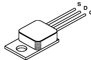
TO-257AA
