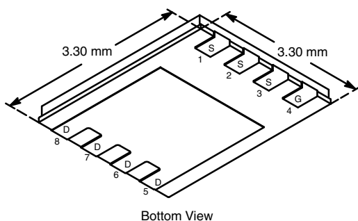
PowerPAK 1212-8
