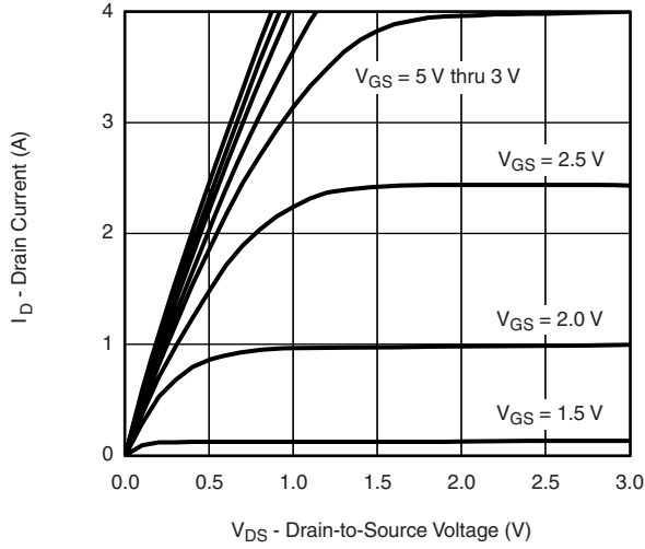
V_{GS} = 5\text{ V thru } 3\text{ V} V_{GS} = 2.5\text{ V} V_{GS} = 2.0\text{ V} V_{GS} = 1.5\text{ V} Output Characteristics
