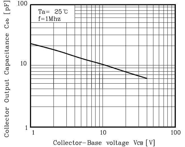
Fig. 10 C_{ob} - V_{CB}
