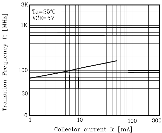
Fig. 11 f_T - I_C
