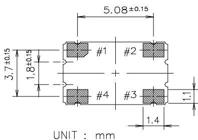
UNIT : mm
