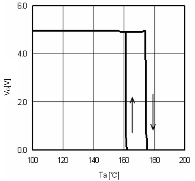
Fig.16 TSD ( I_o=0mA )
