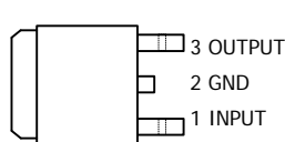
TO-252 3L
