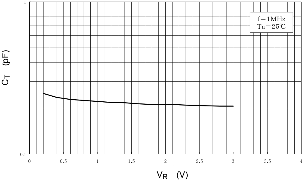
C_T - V_R
