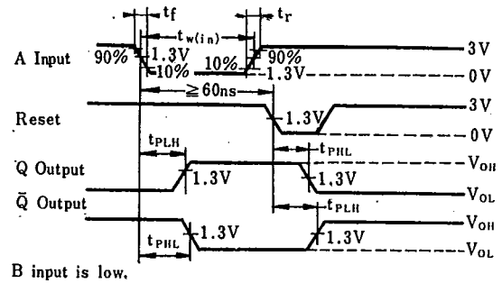
A入力からトリガしてリセットする場合
