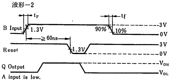
B入力からトリガしてリセットする場合 (2)
