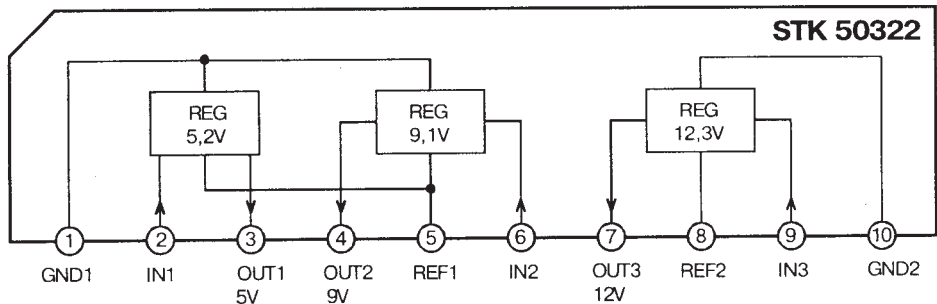
Рис. 3.4. Схема стабилизаторов напряжения источника питания видеомагнитофонов VS-P150EM/EDG (а) и структурная схема микросхемы STK50322(б).
