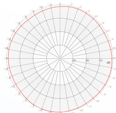
H-plane 3.55 GHz
